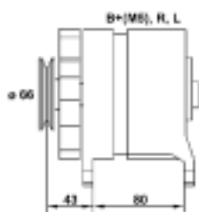
9433 46086 010 MAR6086 40A 14V
