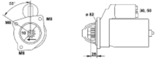
0632 22206 010 MSN618 2,2Kw 12V
