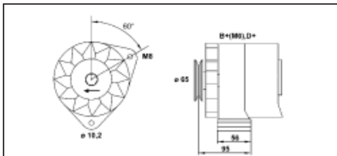
9433 46003 010 MAR6003 70A 14V
