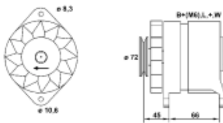
9433 56561 010 MAR962 70A 14V
