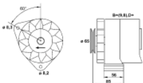
9433 56447 010 MAR475 35A 14V
