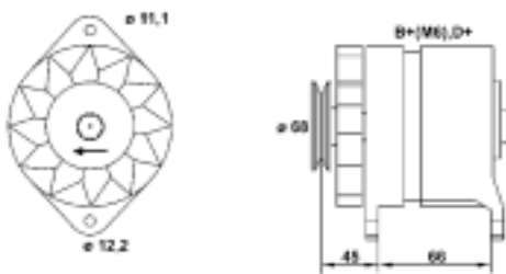
0633 21112 010 MAN379 55A 14V
