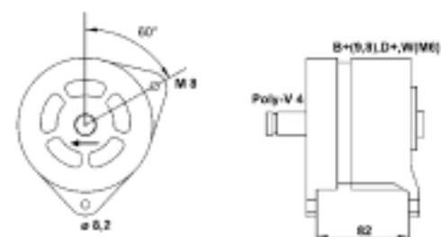
0633 24316 010 MAN160 55A 14V
