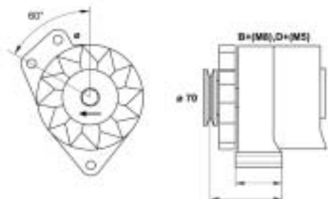
9433 56606 010 MAR508 65A 14V
