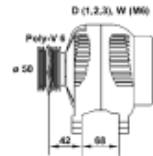
0633 77401 010 MAN7401 80A 14V
