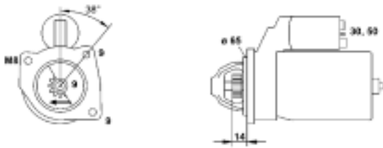
0631 01015 010 MSN829 0,8Kw 12V
