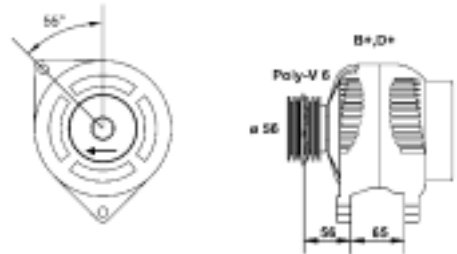
9433 55231 010 MAR5731 95A 14V
