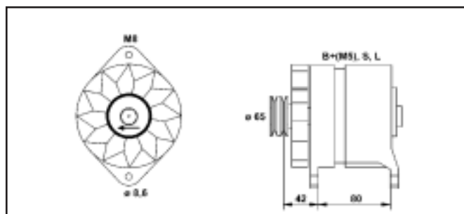
9433 46023 010 MAR6023 50A 14V
