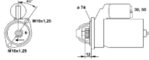
9432 54083 010 MSR2083 0,8Kw 12V
