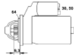
0631 03026 010 MSN403 1,0Kw 12V
