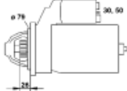
0632 23332 010 MSN626 1,6Kw 12V
