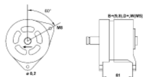
0633 24296 010 MAN155 55A 14V
