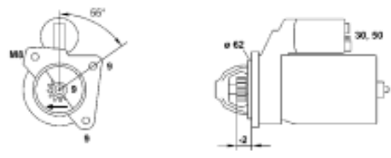
9432 54018 010 MSR2018 1,4Kw 12V
