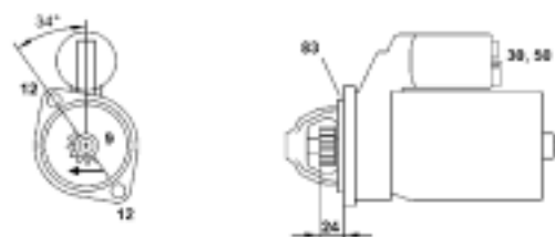
9432 51445 010 MSR427 1,5Kw 12V
