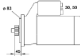
9432 51675 010 MSR495 1,7Kw 12V
