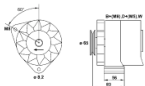
9433 56607 010 MAR509 55A 14V
