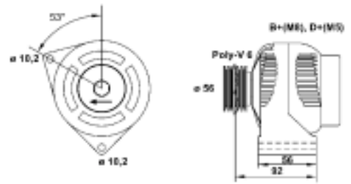
9433 54163 010 MAR7163 70A 14V
