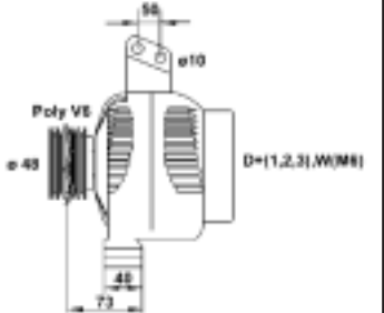
0633 77402 010 MAN7402 80A 14V
