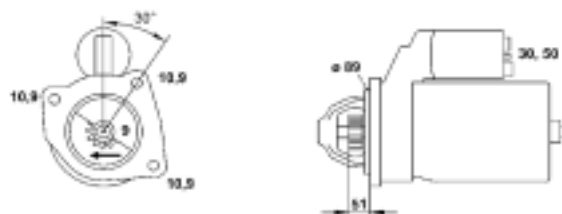
9432 52244 010 MSR726 3,0Kw 12V
