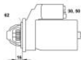
0632 21892 010 MSN314 1,1Kw 12V
