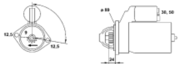
9432 51893 010 MSR933 0,8Kw 12V
