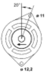
0633 21461 010 MAN868 85A 14V
