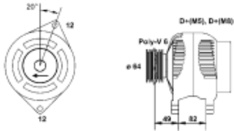
0633 21854 010 MAN955 120A 14V
