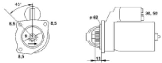
9432 51871 010 MSR515 0,7Kw 12V
