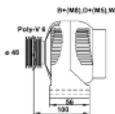
9433 56573 010 MAR969 70A 14V
