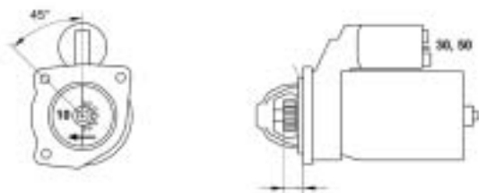
9432 52273 010 MSR734 3,0Kw 12V
