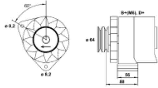
9433 56723 010 MAR599 55A 14V
