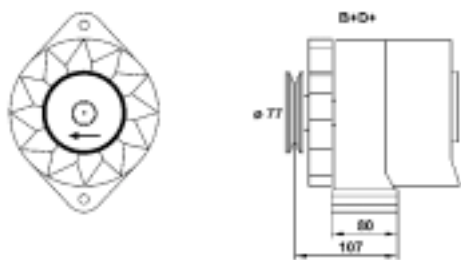
9433 57556 010 MAR895 35A 28V
