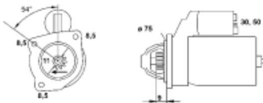
9432 51111 010 MSR367 1,05Kw 12V
