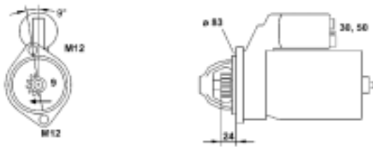
9432 51452 010 MSR669 2,2Kw 12V
