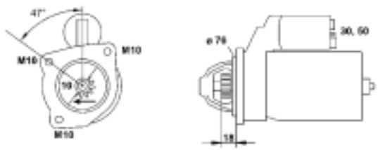
9432 51656 010 MSR484 1,7Kw 12V
