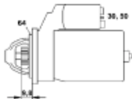
0631 03028 010 MSN404 1,0Kw 12V
