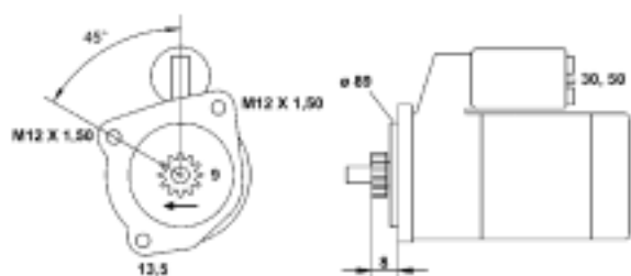
9432 41016 010 MSR1016 2,0Kw 12V
