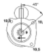
9432 52208 010 MSR701 4,0Kw 24V
